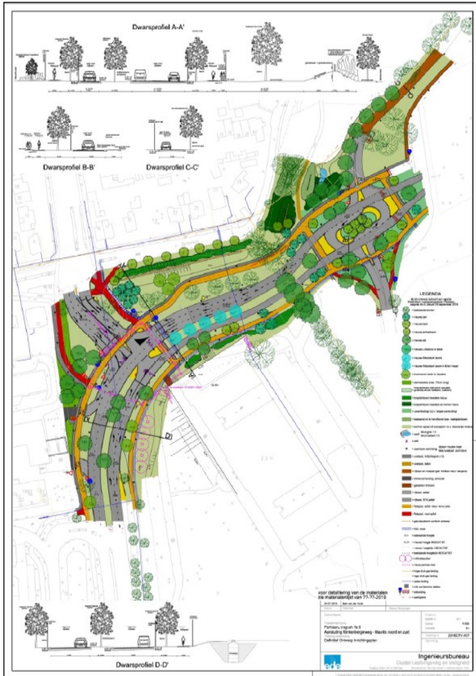
Ontwerp kruispunt 4B5 op tracé Parklaan. Bron: Projectplan Buizerd Nieuwe Kazernelaan te Ede (Natuurbalans - Limes Divergens BV, 2019).
